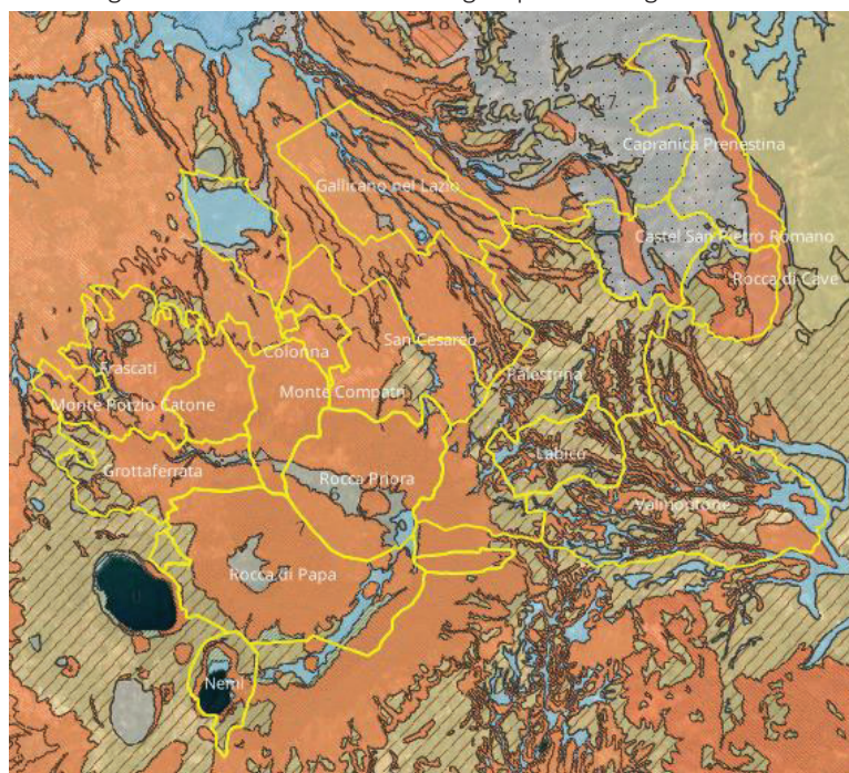
Figura 2 Cartografia geologica dell'area di riferimento GAL
